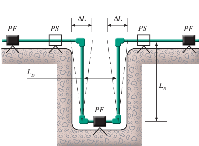
Ejemplo de brazo de compensación en forma de "Ω" Example of "Ω-shaped" compensation arm
