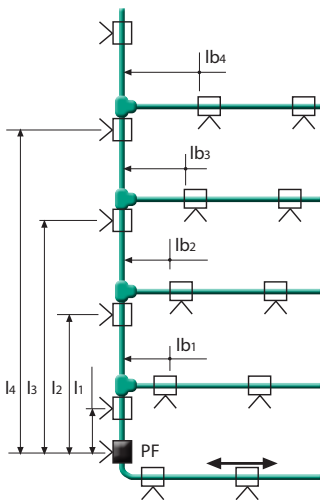
Ejemplo de PUNTO FIJO en tubería vertical. PUNTO FIJO a nivel del suelo.
