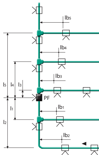
Ejemplo de PUNTO FIJO a nivel intermedio.
